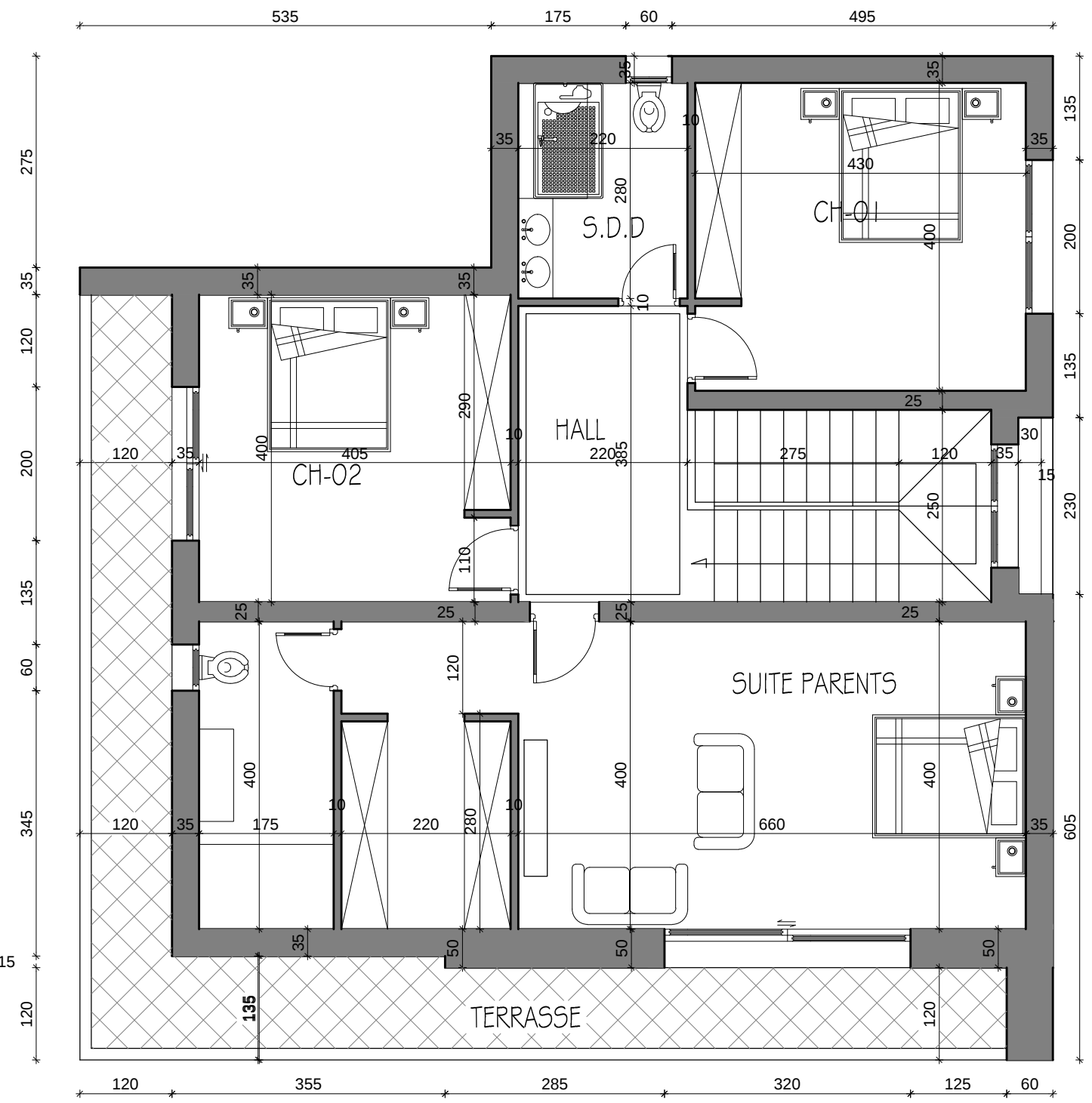
PLAN ETAGE Sc dalle : 150.4 m² Sc habitable : 123.9 m²
