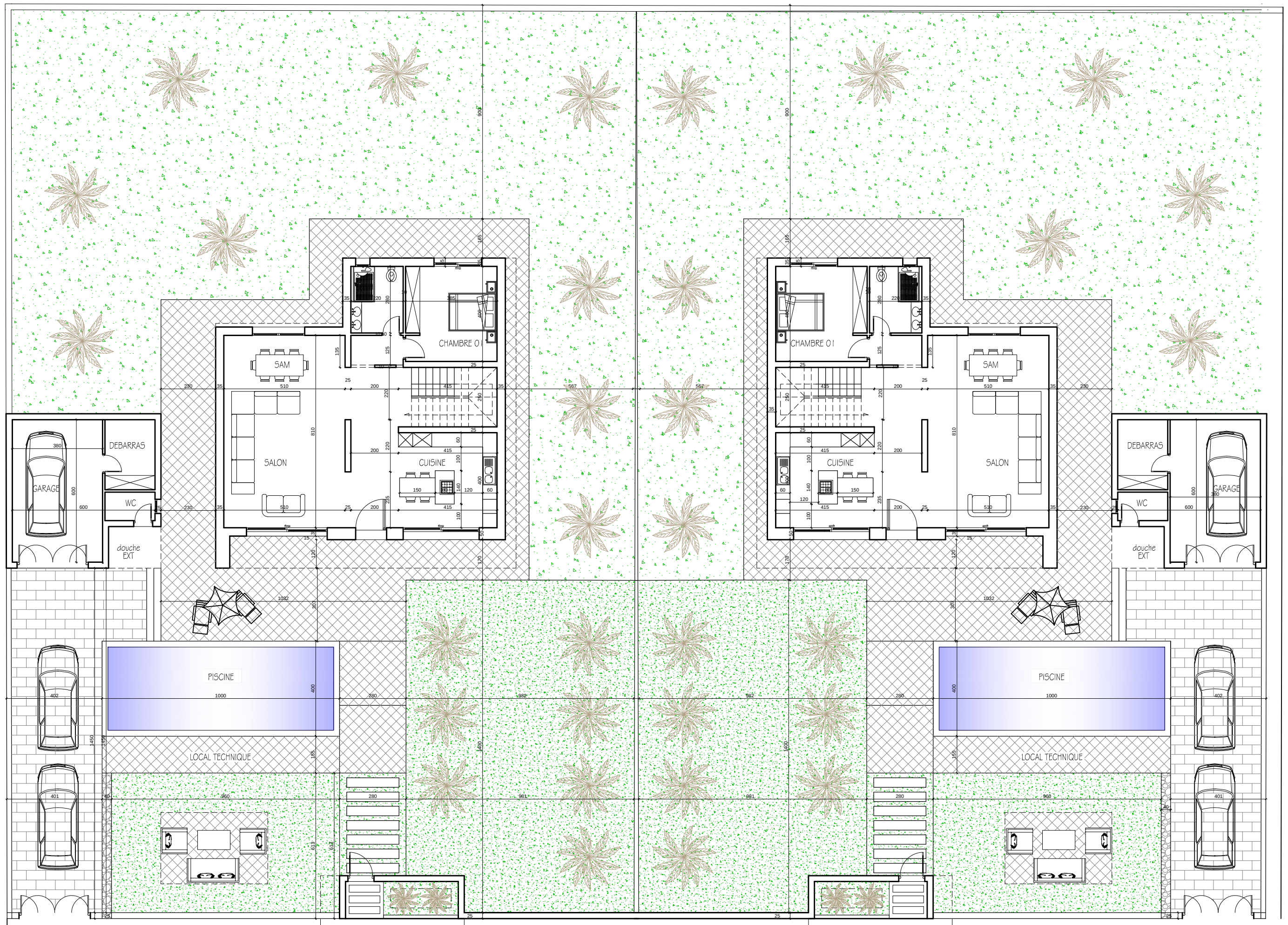
PLAN RDC Sc dalle : 150.4 m² Sc habitable : 129.2 m²
