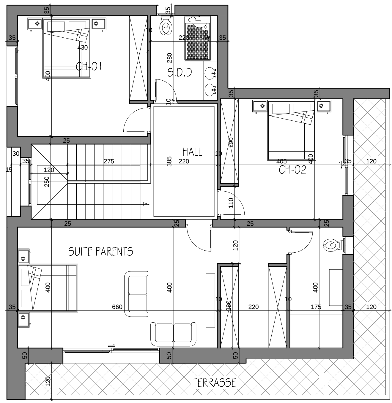
PLAN ETAGE Sc dalle : 150.4 m² Sc habitable : 123.9 m²
